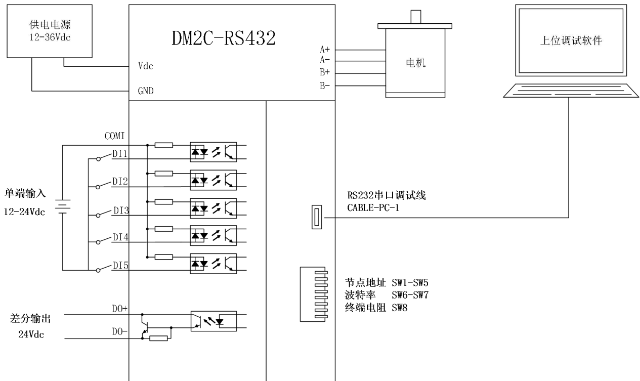
图 3-1 总线步进配线图
