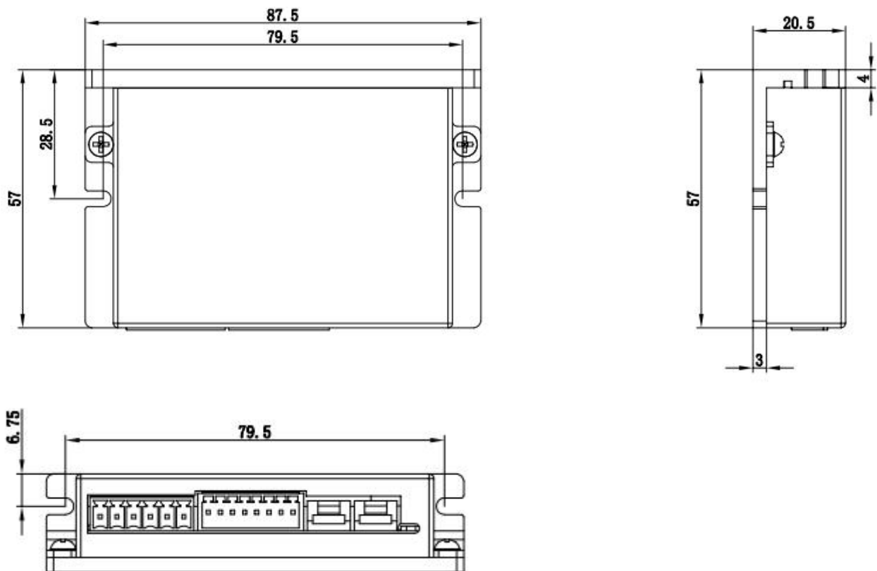
图 2-1 DM2C-RS432 驱动器机械尺寸
