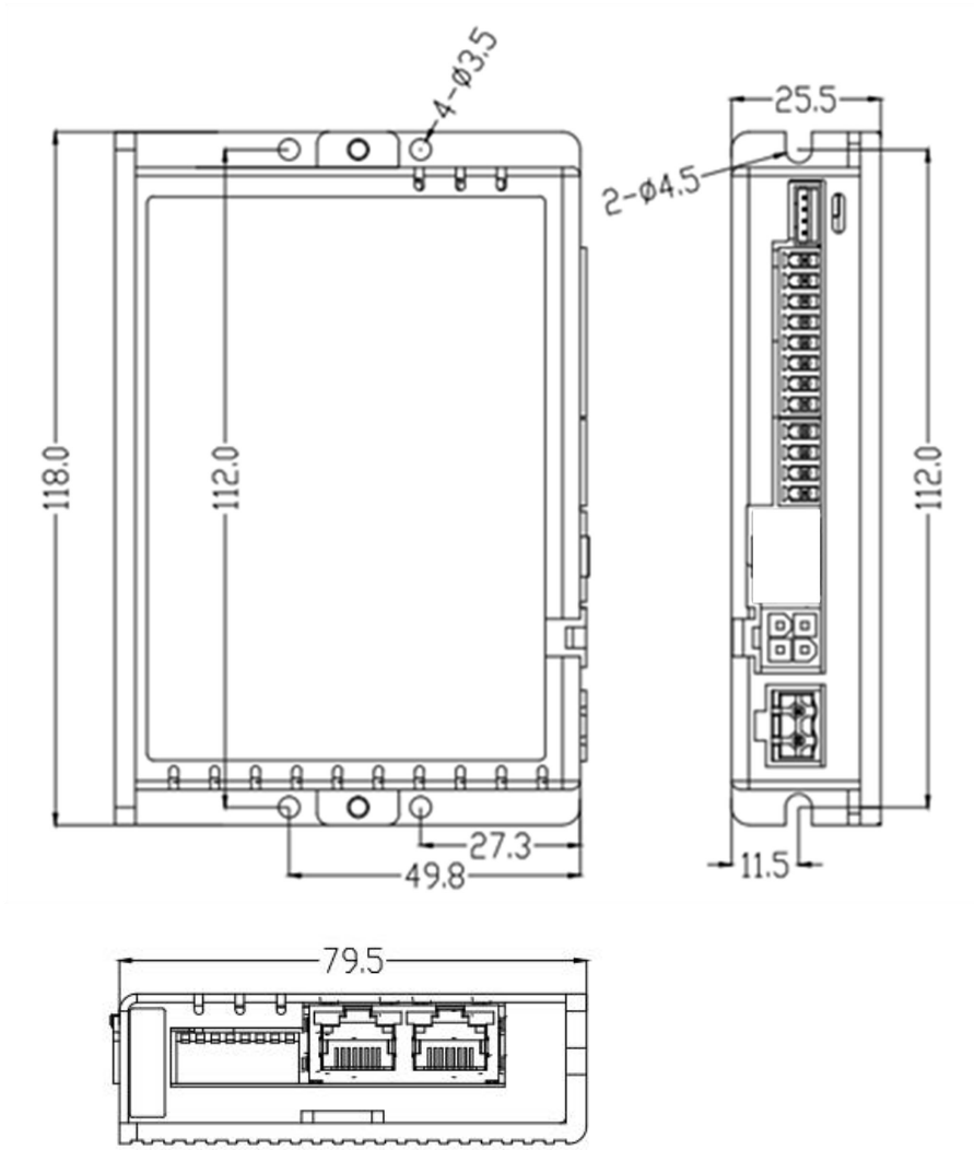
图 2-1 DM2B-RS522/542/556/570 系列驱动器机械尺寸
